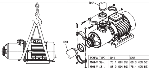
Fig. 7 Sollevamento pompa Raising the pump Anhebung Pumpe Suoèvement de la pompe Elevación de la bomba 吊起水泵
