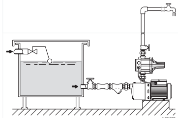
Fig. 1 Funzionamento sotto battente Positive suction head operation Zulaufbetrieb Fonctionnement en charge Funcionamiento bajo carga 正吸上水头的操作
