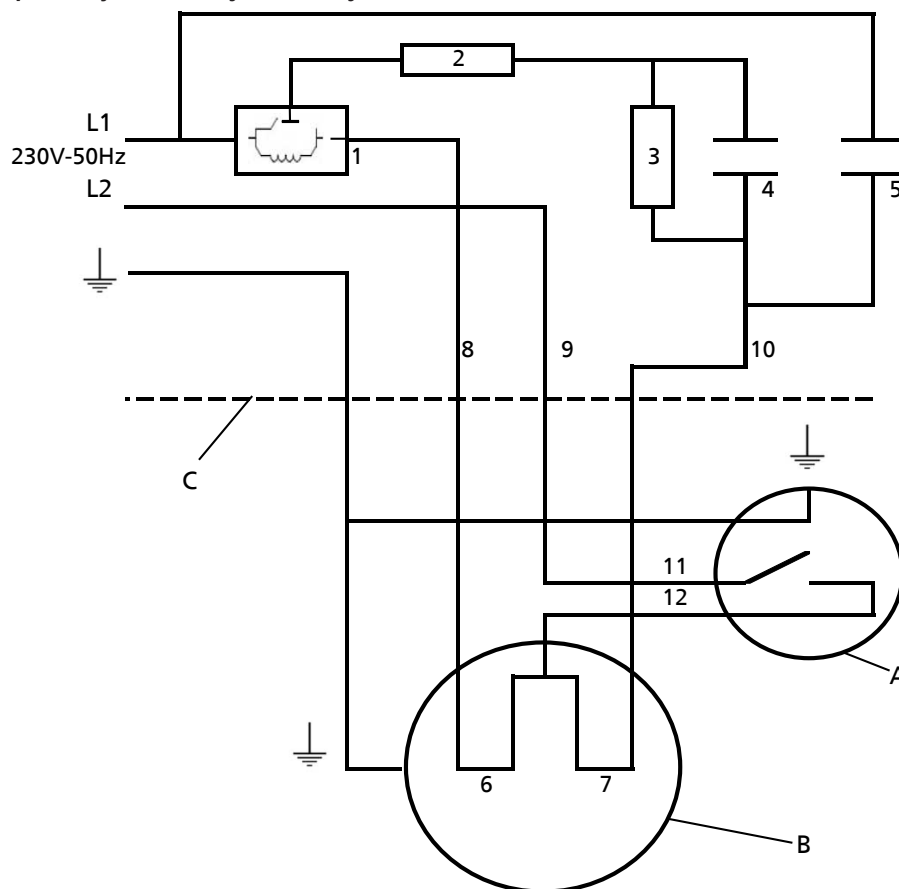
Obr. 22: Provedení na jednofázový střídavý proud s plovákovým spínačem (SE)
