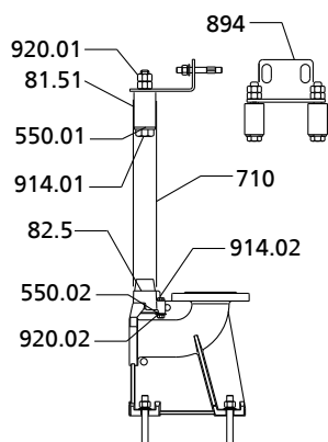
Obr. 10: Montáž 2 vodicích trubek
