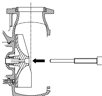
Obr. 19: Odtlačovací šroub
