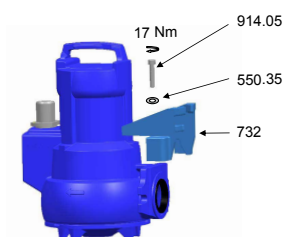
Obr. 12: Montáž třmenového vedení
