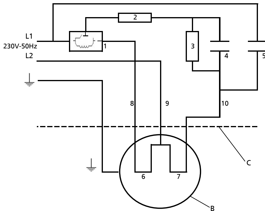
Obr. 23: Provedení na jednofázový střídavý proud bez plovákového spínače (NE)
