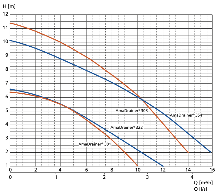
Charakteristiky AmaDrainer® 3
